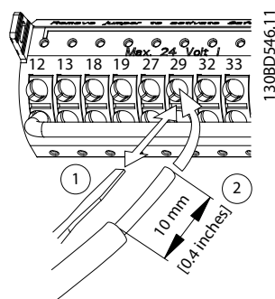
Ilustracja 5.21 Podłączanie elastycznych (linkowych) przewodów sterowania
