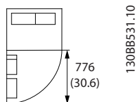
Disegno 3.4 Spazio davanti a custodie con protezione IP21/IP54, grandezza telaio F8
