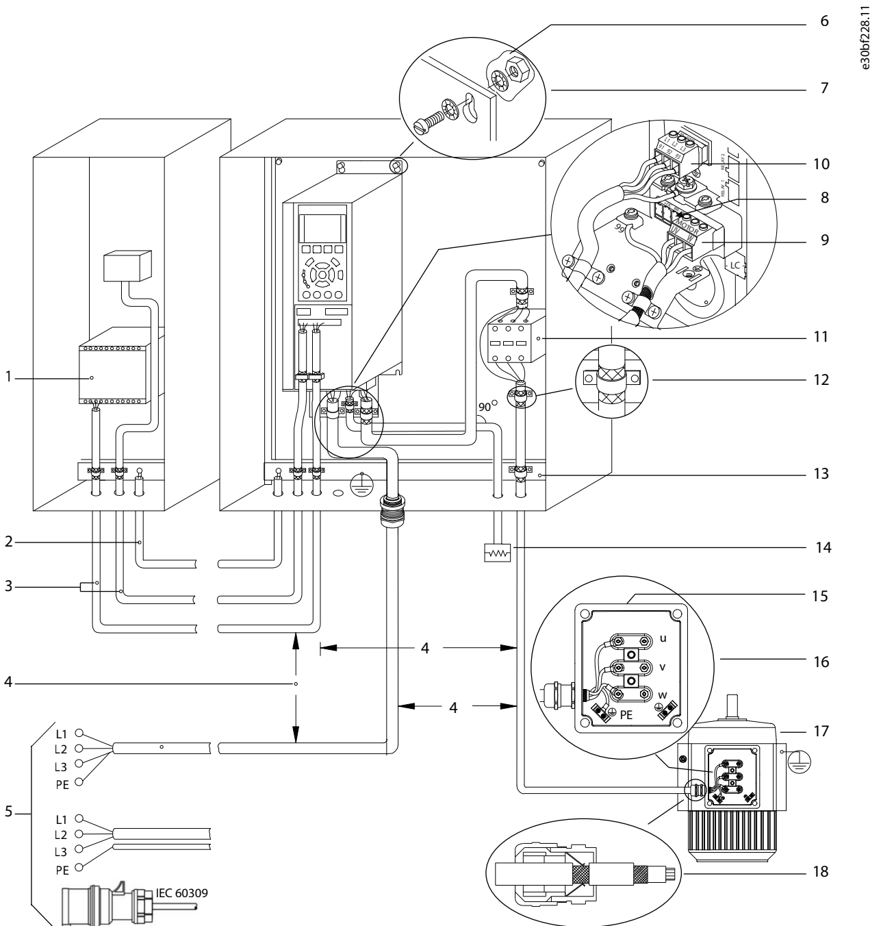
Illustrazione 17: Esempio di installazione EMC corretta
