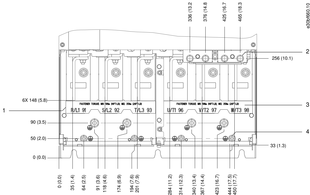
Illustrazione 26: Dimensioni dei morsetti E3h (vista frontale)
