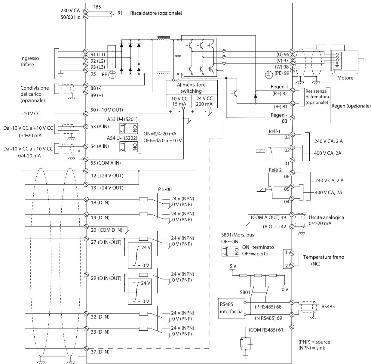
Illustrazione 18: Schema di cablaggio di base
