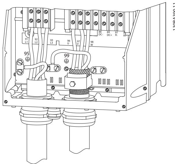
Ilustracija 4.8 Kabli motorja, napajanja in ozemljitve za ohišja tipov B in C (izolirani kabli)
