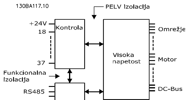
Ilustracija 8.1 Izolacija PELV
