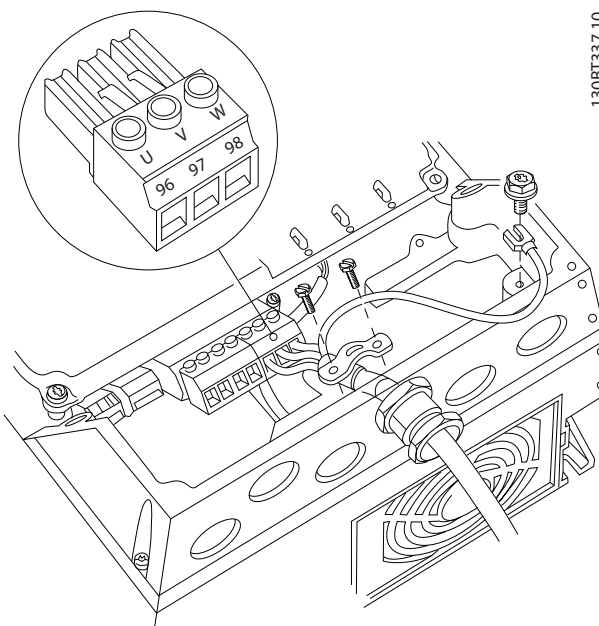
Ilustracija 4.7 Vezava motorja za tipe ohišja A4/A5 (IP55/66/ NEMA tip 12)
