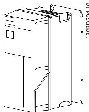
Εικόνα 3.3 Σωστή τοποθέτηση με πίσω πλάκα
