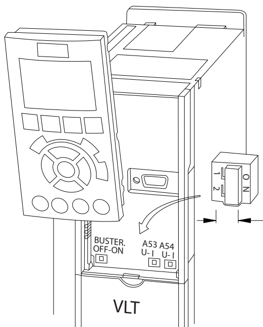
Εικόνα 4.16 Τοποθεσία διακοπών ακροδεκτών 53 και 54
