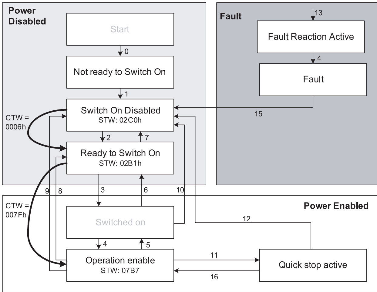
Disegno 6.6 Macchina a stati DSP 402
