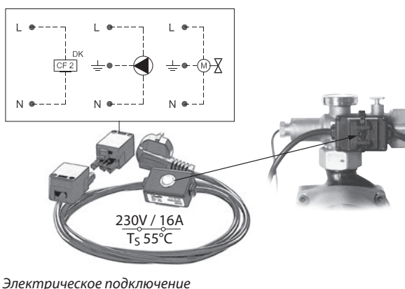
Электрическое подключение
