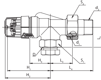
Yatay açılı vana RA-FN
