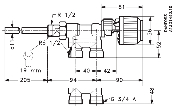
Side connection 1/2" und 3/4"
