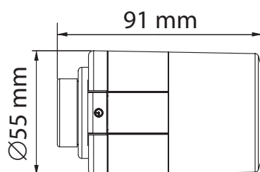
avec l'adaptateur de vanne M28
