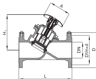
DN = 80–150 мм
