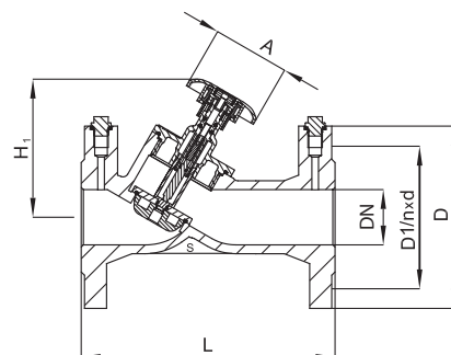
DN = 15–50 мм
