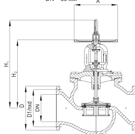
DN = 200–400 мм
