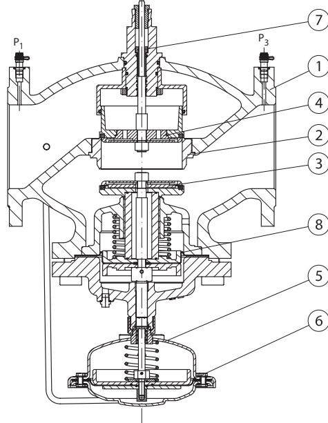
DN = 150 мм
