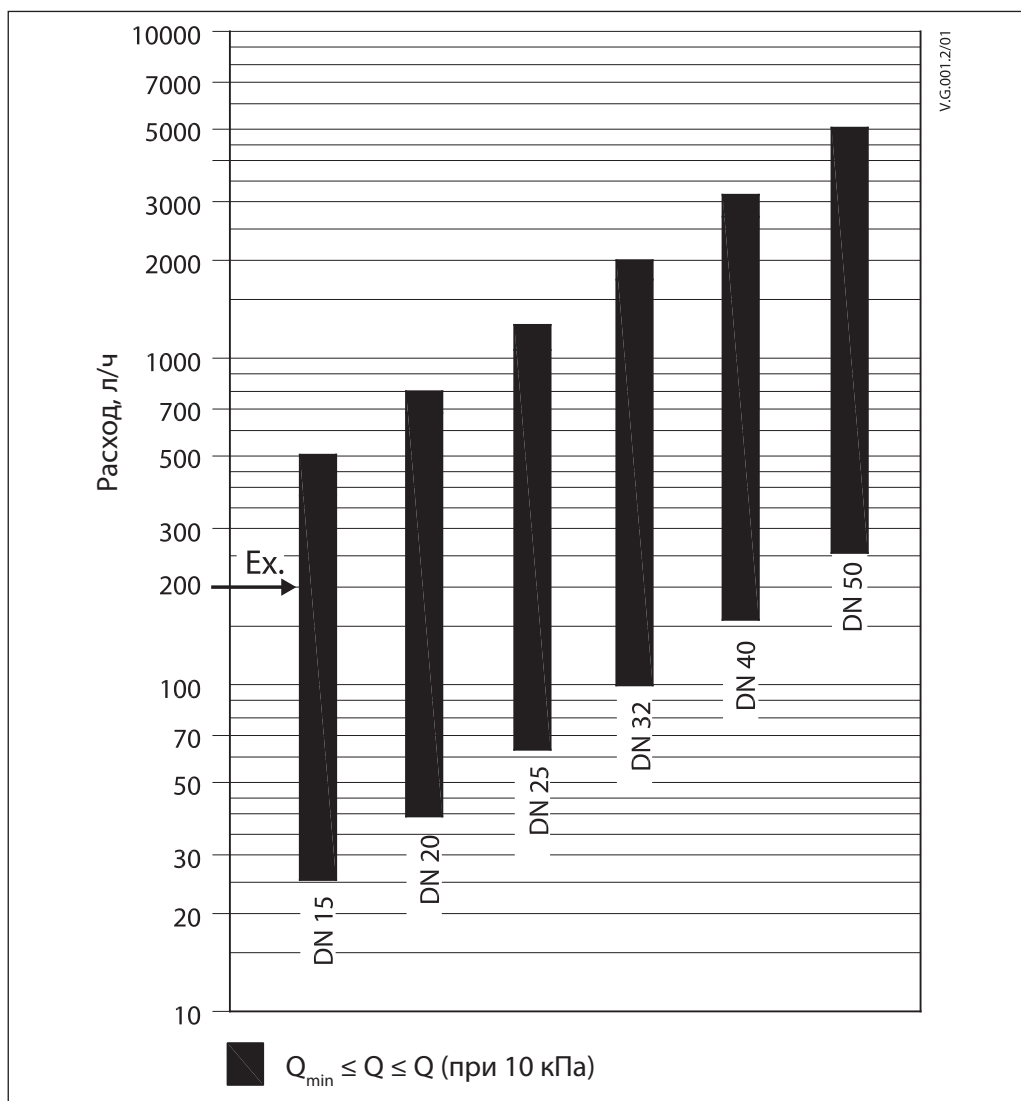
Диаграмма подбора клапана АРТ при ΔP БК = 10 кПа
