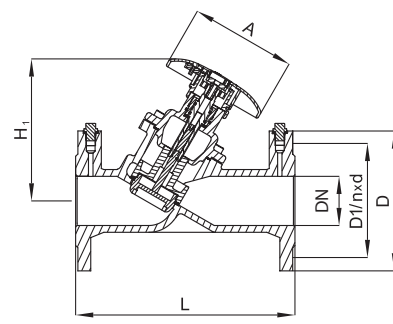
DN = 65 мм
