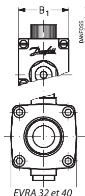
EVRA 32 et 40 Bobina con caja terminal
