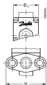
EVRA 25 Bobina con caja terminal
