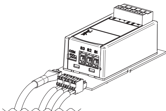
Sensor de entrada e montagem do cabo de comunicação (a imagem mostrada é para EETa 3W)
