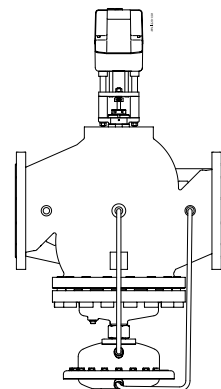
AFQM PN 16 DN 150-250 + AMV(E) 85/86
