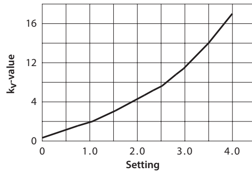
Akış karakteristikleri
