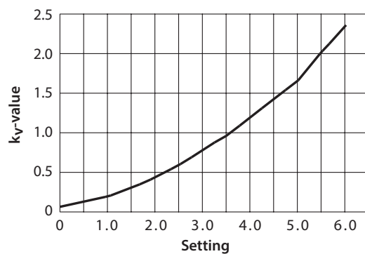
Flödeskaraktistik
