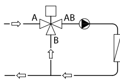
Fig. 2: Vană de amestec utilizată în aplicații de amestec
