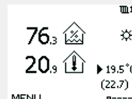
Наприклад, головний екран 1 в А230.3, де відображається мінімально необхідна температура приміщення (22,7):
