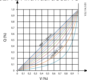
AV:4 / 32772 Alfawaardecurve
