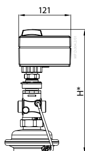
AMV(E) 10 + AVQM (DN 15)
