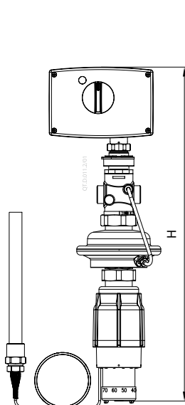
STM / AVQMT / AMV(E) + AVQM (DN 15-50)
