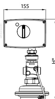
AMV(E) 2./3. + AVQM (DN 15-50)
