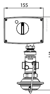
AMV(E) 2./3. + AVQM (DN 15-32)
