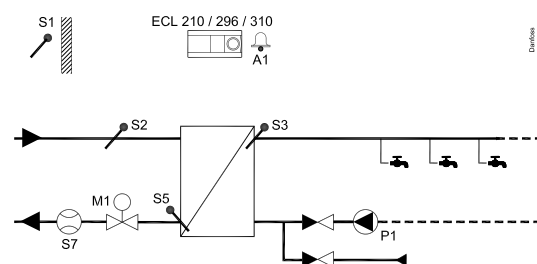
Typowa aplikacja A217.3, przykład a:
