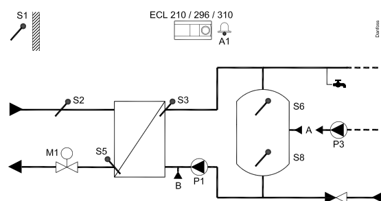
Typowe zastosowanie aplikacji A217.1/A317.1:
