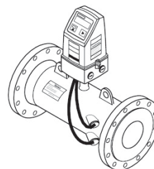
Cableado al caudalímetro SONO 3500CT:
