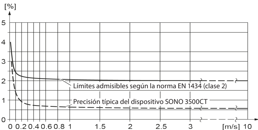
Precisión de la medición según la Directiva MID (clase 2)
