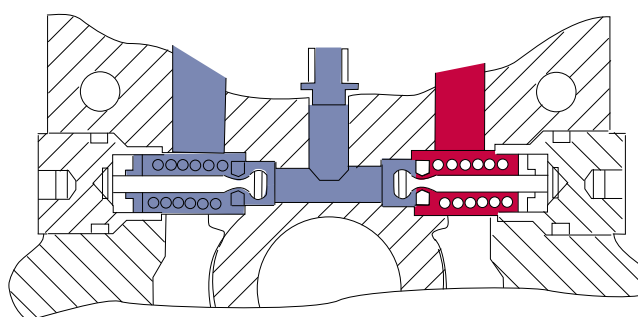
HPRV valve
