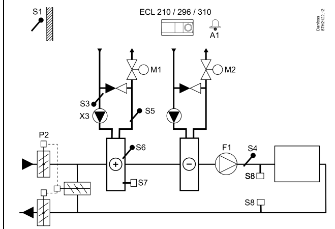
Typisk A214.4-applikation:
