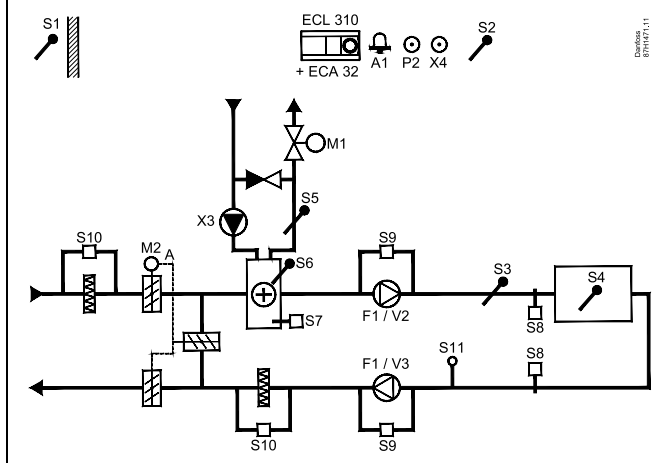
Typisk A314.9-applikation:
