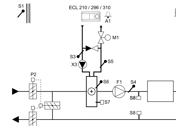
Typisk A214.2-applikation:
