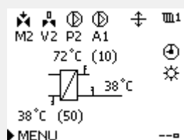
Příklad zobrazení displeje s indikací vlivu:
