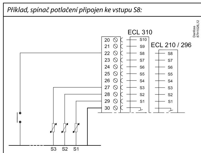
Příklad, relé potlačení připojeno ke vstupu S8:
