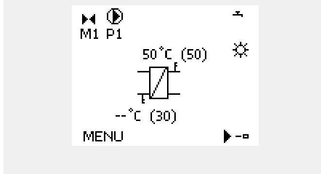
Příklad zobrazení s tepelným výměníkem:
