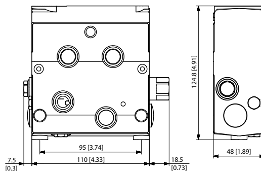
PVSP – Abmessungen
