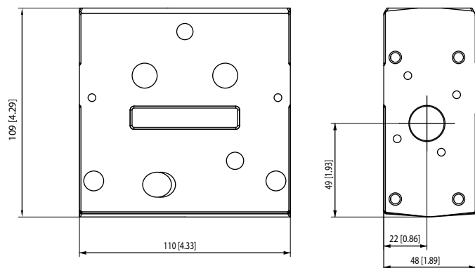
PVSKM-Modulabmessungen
