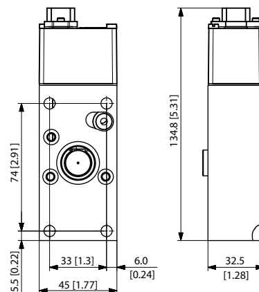
Abmessungen PVDI-Richtungsanzeige
