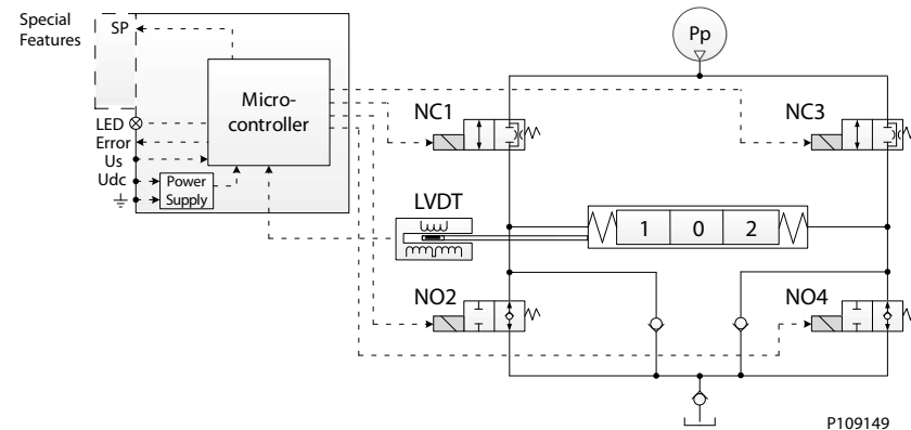
PVES-SP-Funktionsdiagramm
