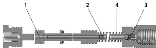
Schnittzeichnung Kompensatorschieber
