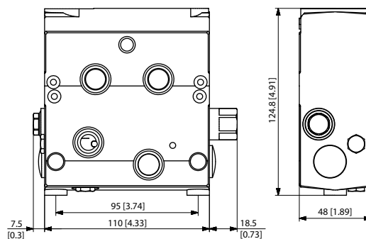
PVSPM – Abmessungen
