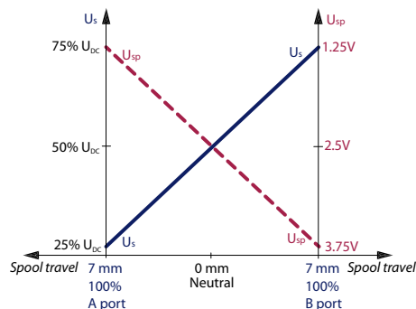
Feedback Schieberposition
