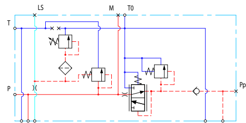
Open-Center-PVP mit PPRV und T0
