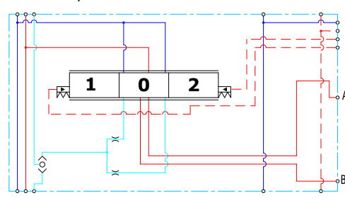
Nicht kompensiertes PVB mit T0
