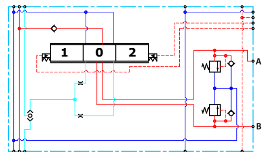
Nicht kompensiertes PVB mit Lastabfall-Rückschlagventil und T0
