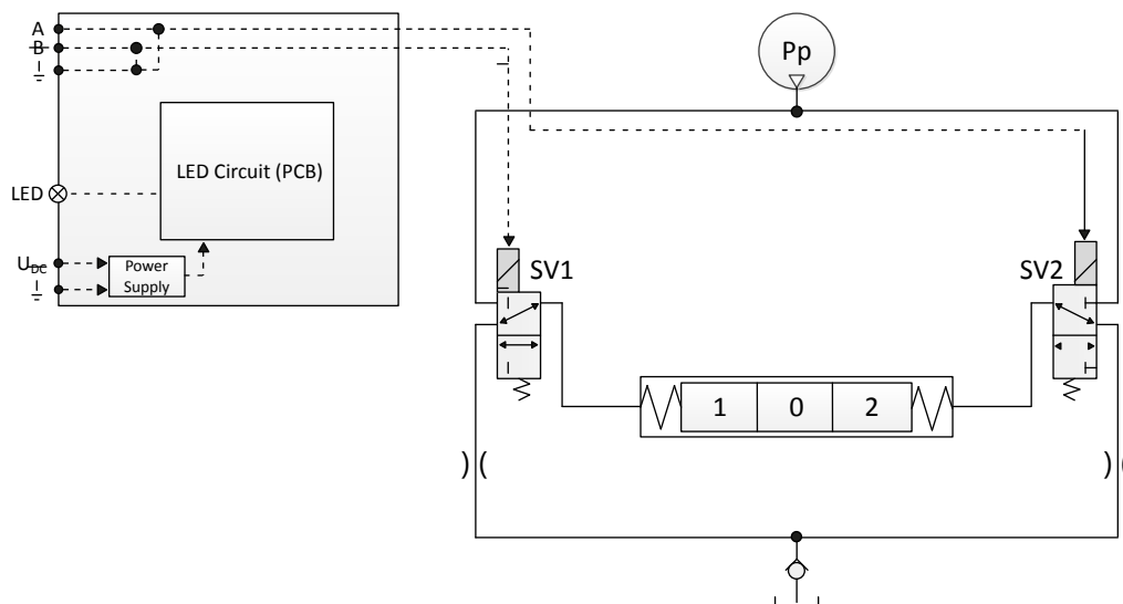
PVEO 功能图
