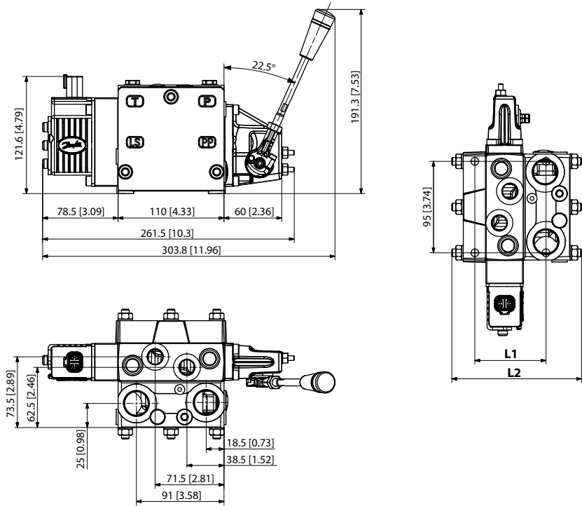
PVB 16 尺寸（12 联）
