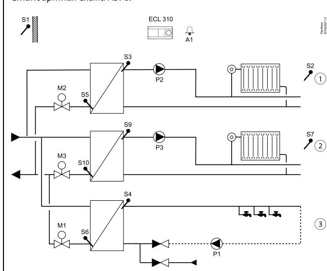
Стандартная схема A376:
