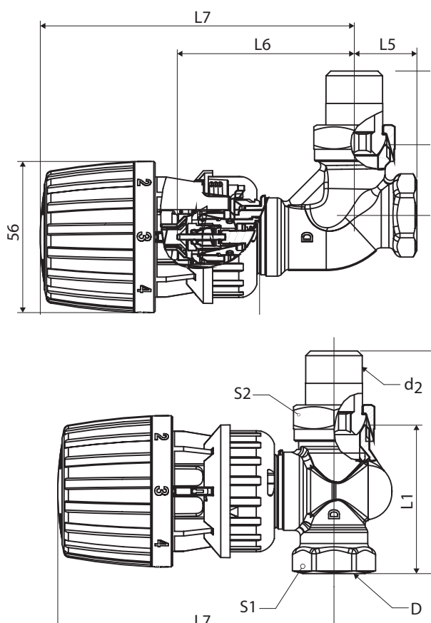
RA-DV DN 20 Durchgangs- und Eckventil/Fühler RA 2990
