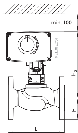
AMV(E) 438 SU + VF 2 (DN 15 – 50) AMV(E) 25 (SU/SD), 35 + VF 2 (DN 15 – 50) + adaptor 065Z0311
