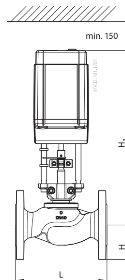
AMV(E) 56 + VF 2 (DN 65 – 80) + adaptor 065Z0312
