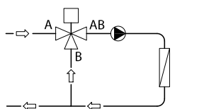
Slika 2: Mešalni ventil, ki se uporablja v mešalni aplikaciji
