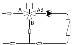
2. att. Jaukšanas vārsts, kas tiek izmantots jaukšanas pielietojumā
