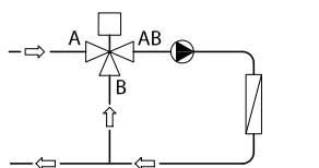
2 pav. Srautams maišyti naudojamas maišymo vožtuvas
