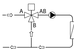
Fig. 2: Válvula de mezcla usada en una aplicación de mezcla
