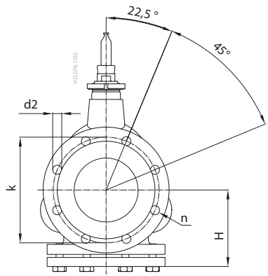
VF 2 (DN 125, 150)
