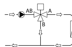
Fig. 4: Válvula diversora usada en una aplicación de desvío
