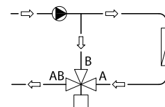
Fig. 3: Válvula de mezcla usada en una aplicación diversora
