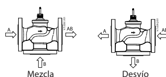
Fig. 1: Conexión de mezcla o desvío
