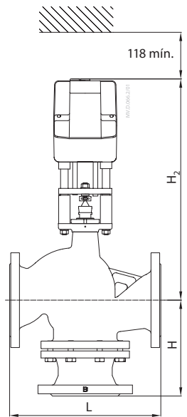
AMV(E) 85, 86 + VF 2 y VF 3 (DN 125, 150)
