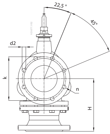
VF 3 (DN 125, 150)
