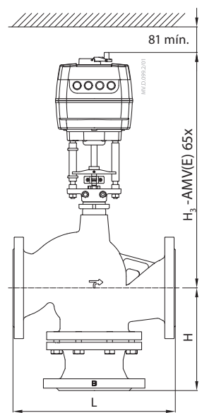
AMV(E) 65x + VF 2 y VF 3 (DN 125, 150)
