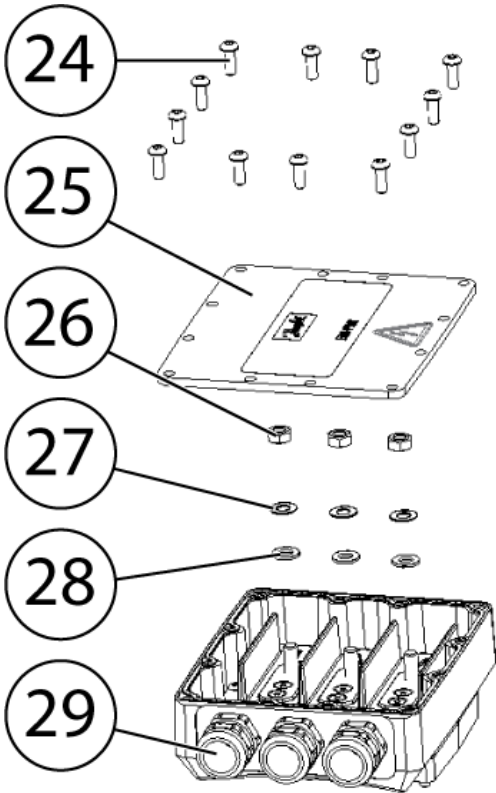
高压接头装配结构
