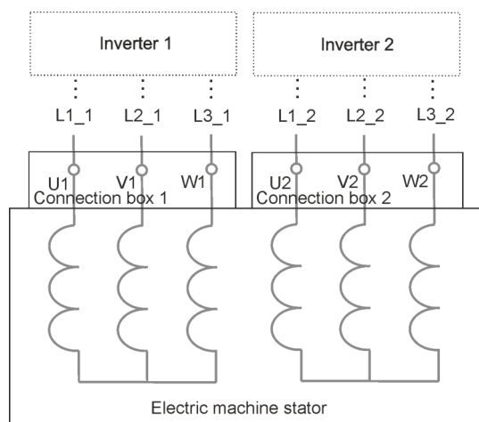
DUAL 选件的接线图
