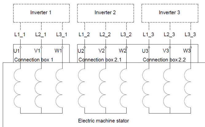
TRI 选件的接线图
