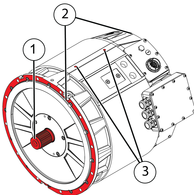
电机的机械安装接头（水平安装）
