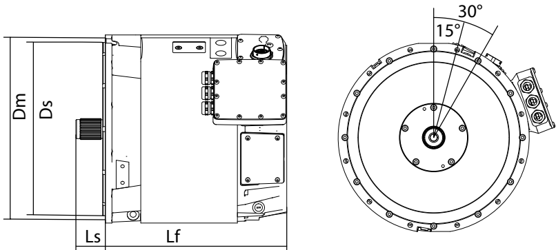
电机的主要尺寸
