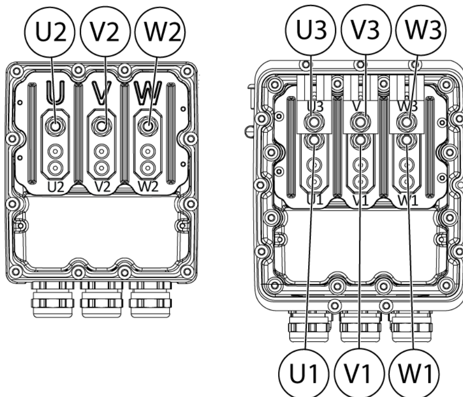
TRI 选件接线点
