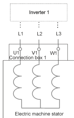
SINGLE 选件的接线图
