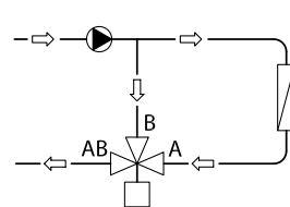
Slika 3: Mešalni ventil, ki se uporablja v delilni aplikaciji
