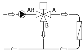
Joonis 4 Jagamisventiil jagamisrakenduses
