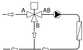
Joonis 2 Segamisventiil segamisrakenduses
