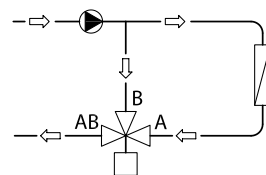
Joonis 3 Segamisventiil jagamisrakenduses
