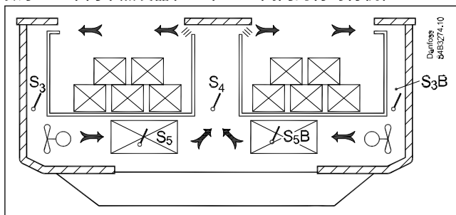
数字 23: 带两个蒸发器和一个 AKV 阀门的背对背机柜
