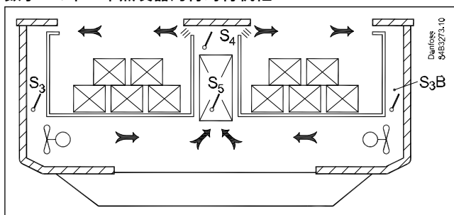
数字 22: 带一个蒸发器的背对背机柜
