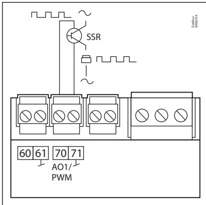
数字 38: 用于防露加热的外部固态继电器
