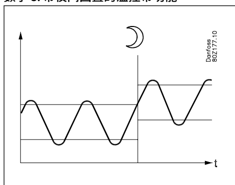
数字 8: 带夜间回置的温控带功能
