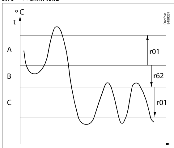
数字 19: 加热功能
