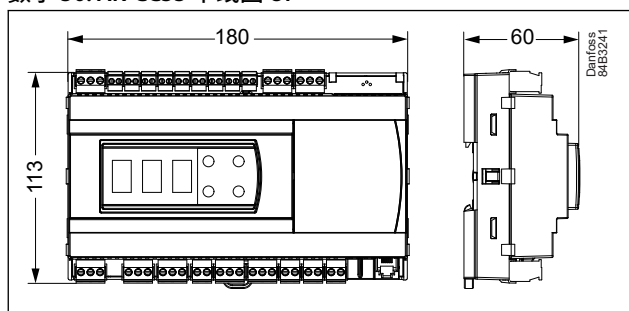
数字 50: AK-CC55 单线圈 UI
