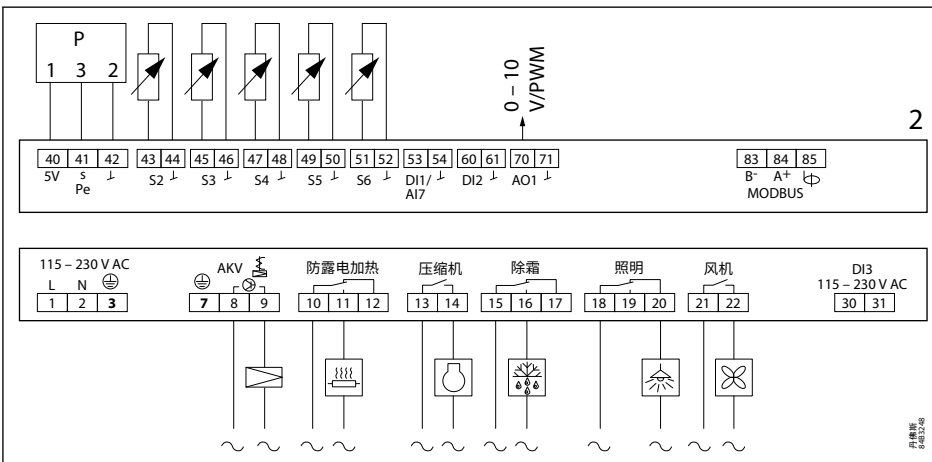
数字 27: 应用 2 的连接
