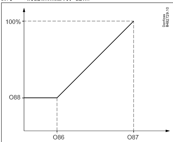
数字 14: 防露加热控制, 露点
