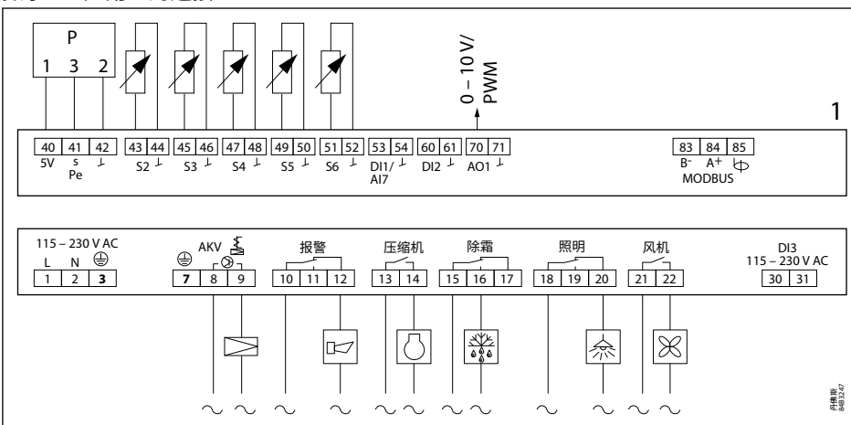
数字 27: 应用 2 的连接
