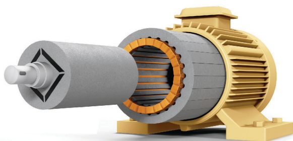
PM-Motor mit vergrabenen Magneten
