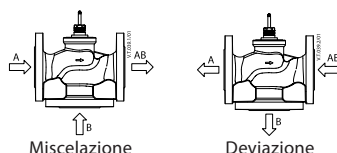
Fig. 1: Collegamento in miscelazione o deviazione
