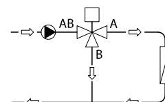
Fig. 4: Valvola deviatrice utilizzata in applicazioni di deviazione
