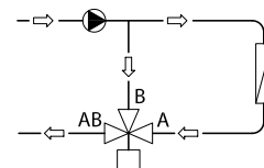
Fig. 3: Valvola miscelatrice utilizzata in applicazioni di deviazione
