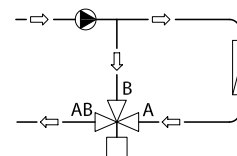
Obrázok 3: Zmiešavací ventil používaný pri rozdeľovacích aplikáciách
