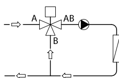
Obrázok 2: Zmiešavací ventil používaný pri zmiešavacích aplikáciách
