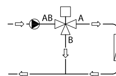
Obrázok 4: Odberový ventil používaný pri rozdeľovacích aplikáciách
