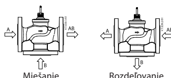
Obrázok 1: Spoj miešania alebo rozdeľovania
