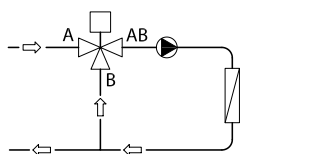
Bild 2: Blandningsventil använd i en blandningstillämpning
