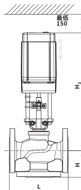
AMV(E) 56 + VF 3 (DN 65-80) + 适配器 065Z0312
