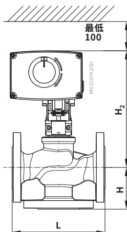
AMV(E) 438 SU + VF 3 (DN 15-50) AMV(E) 25 (SU/SD), 35 + VF 3 (DN 15-50) + 适配器 065Z0311
