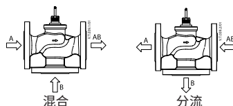
图 1: 混合或分流连接
