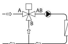
图 2: 合流阀 (混合应用)
