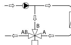
图 3: 合流阀 (分流应用)
