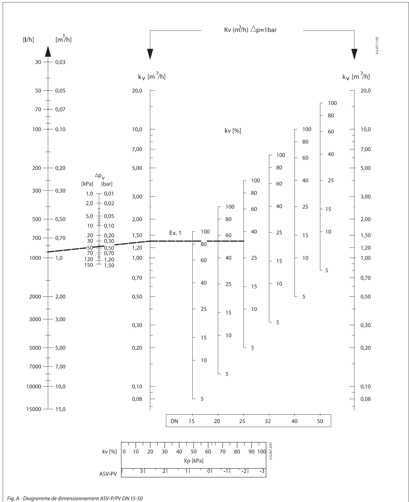
Fig. A - Diagramme de dimensionnement ASV-P/PV DN 15-50
