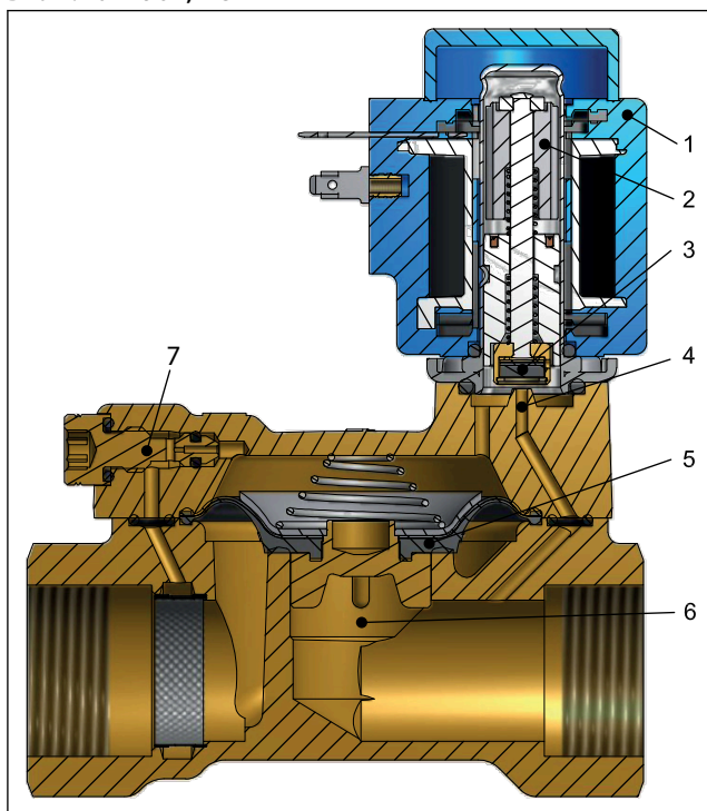
Bild 2: Funktion, NO
