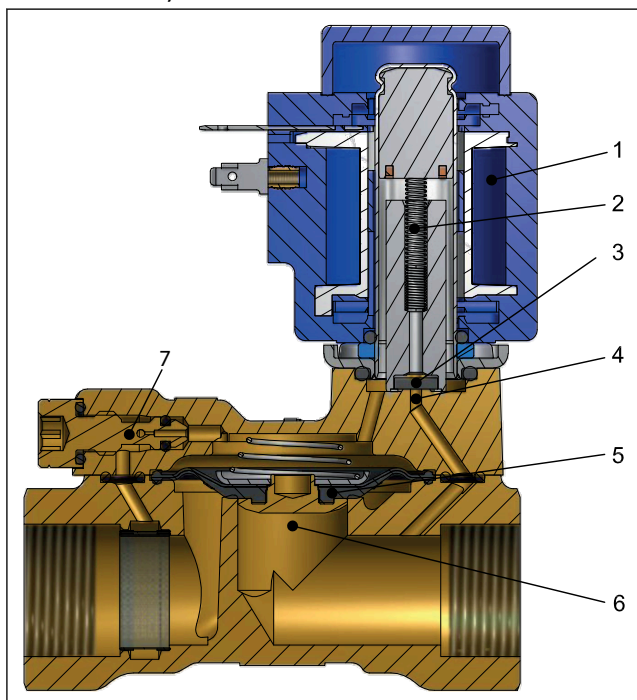
Bild 1: Funktion, NC
