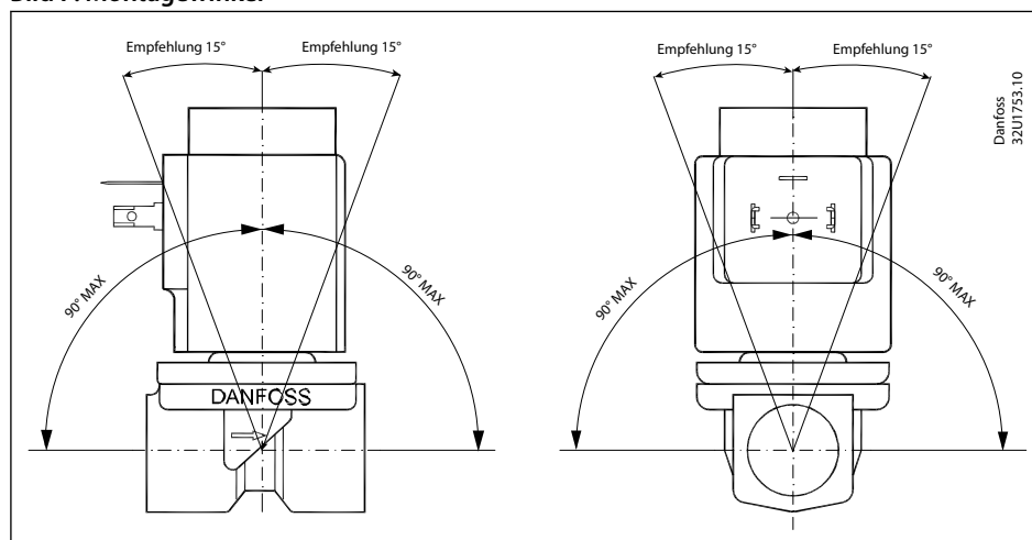
Bild 7: Montagewinkel
