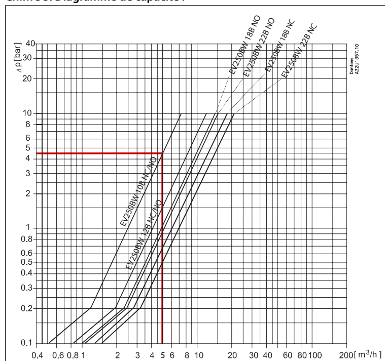
Chiffre 5: Diagramme de capacité :
