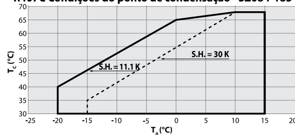
R407C Condições do ponto de condensação - SZ084-185
