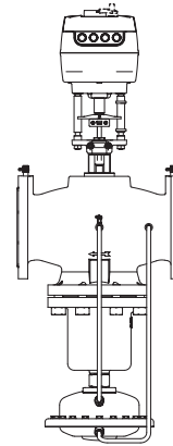
NovoCon® L / SU / SD AB-QM DN 125 - 150HF
