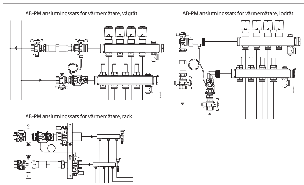
Figur 4) AB-PM-anslutningssats för fördelningsledning (vågrät eller lodrät anslutning)
